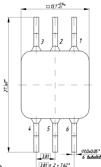
2М420А4: исполнение 4 (поверхностный монтаж):
