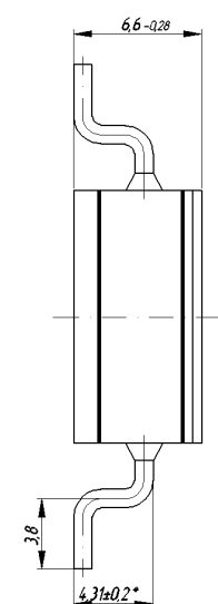
2М420А4: исполнение 4 (поверхностный монтаж):
