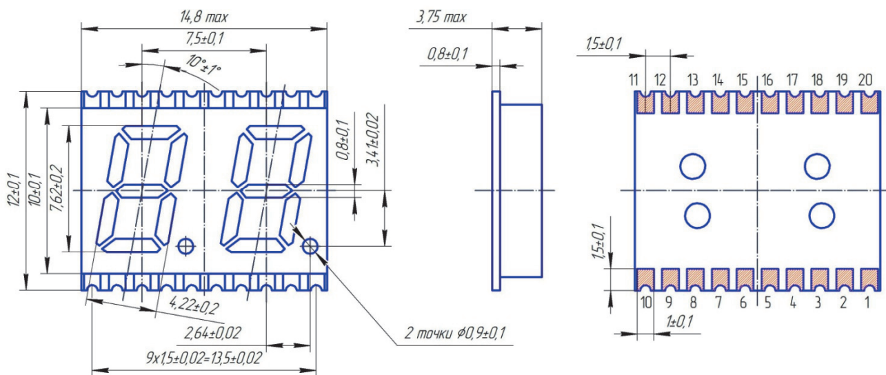
Двухразрядный индикатор
