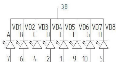
Схема включения с общим катодом (ИПЦ53А91-1/7)
