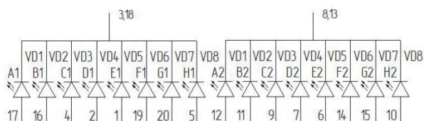
Схема включения с общим катодом (ИПЦ54A91-2/7)
