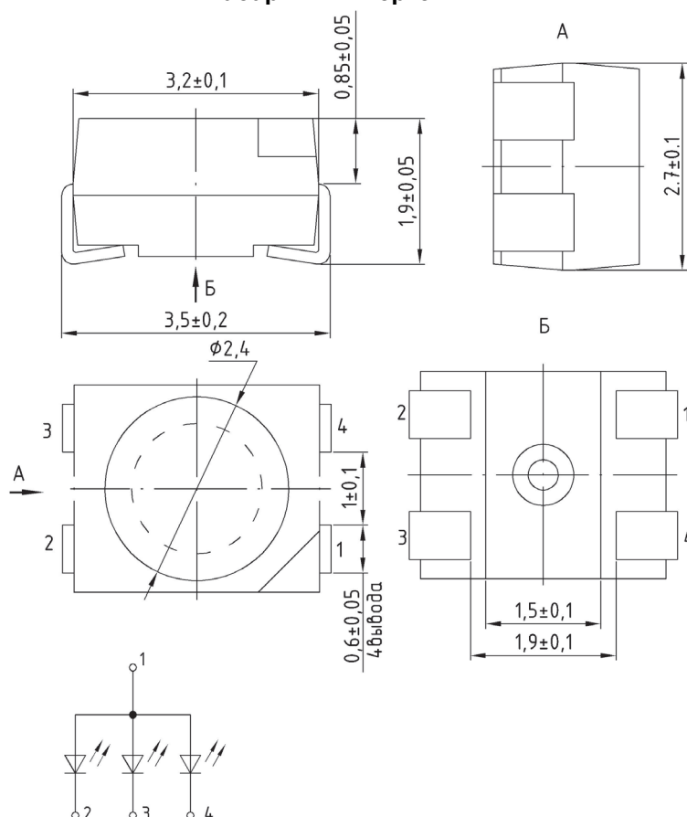
Габаритный чертеж
