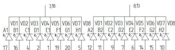
Схема включения с общим катодом (ИПЦ53А9-2/7)
