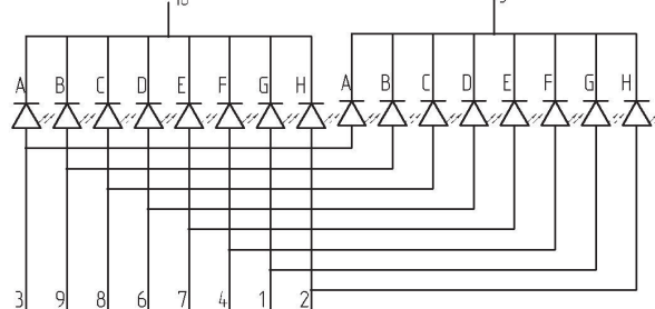
Схема электрическая с общим катодом
