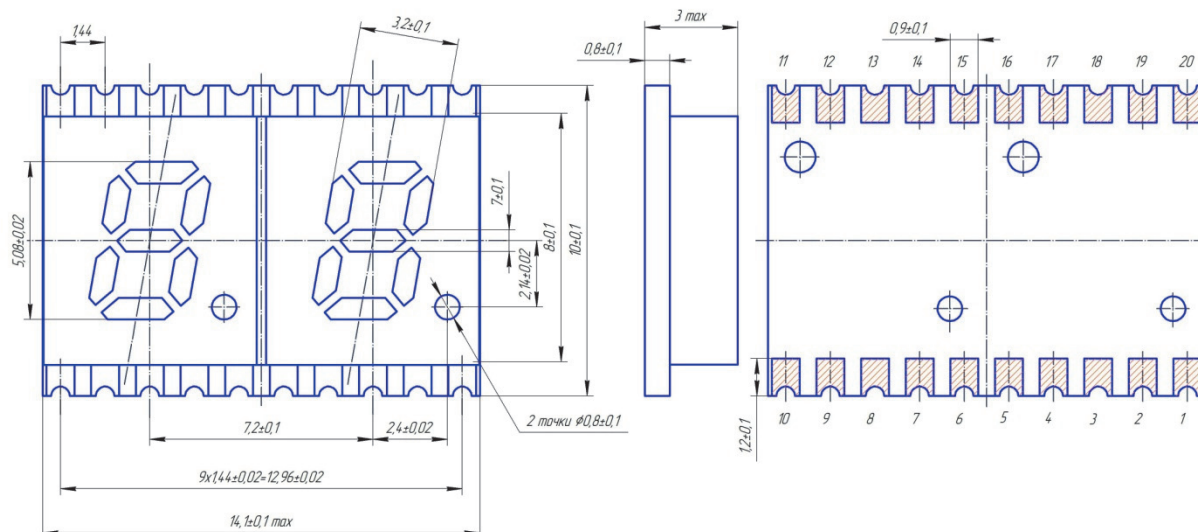
Двухразрядный индикатор
