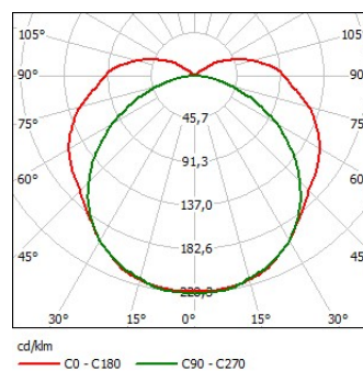
A - cosine Plant-50-ABC
