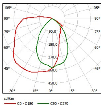
A - cosine Plant-30-ABC
